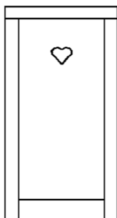
Type N Panneau complet de 22 mm
